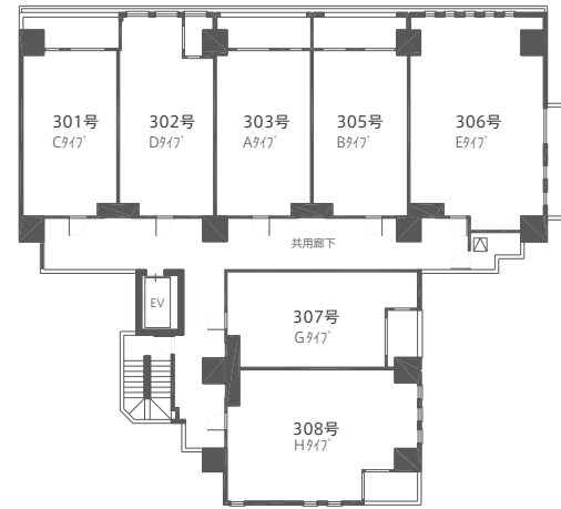
3F平面図
